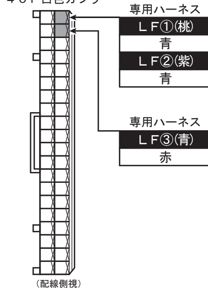
ヒューズブロック裏側の 右上側 40P白色カプラ
