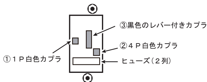
【BCM&J/B正面拡大図】
