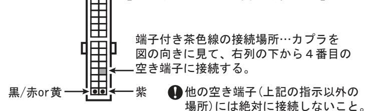
【カプラ…ハーネス側より見た図】
