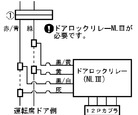
車両室内側
