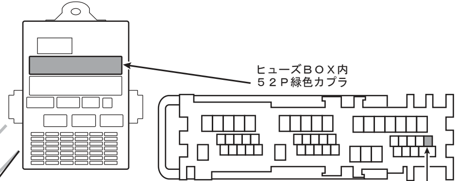
ヒューズBOX表拡大図
