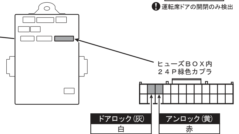
ヒューズBOX裏拡大図
