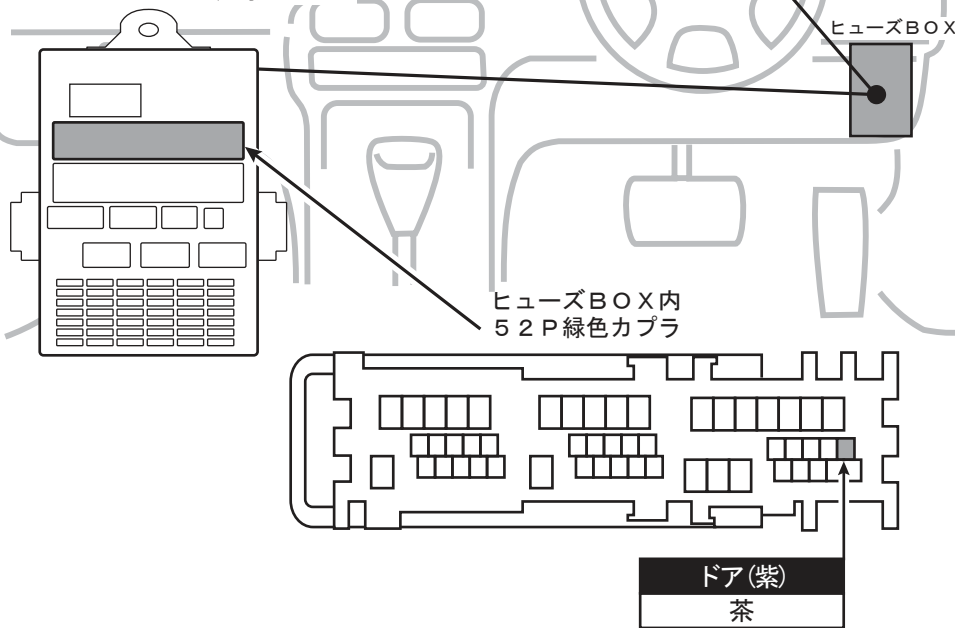
ヒューズBOX表拡大図
