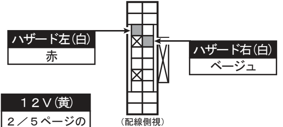
ヒューズブロック内左側 18P 黒色カプラ
