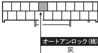
スマートキーECU 3個並んでいる一番左側 20P灰色カプラ
