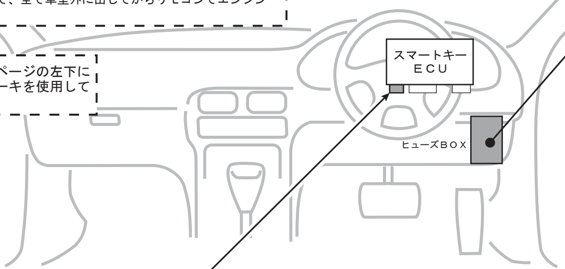
スマートキーECU 3個並んでいる一番左側 20P灰色カプラ
