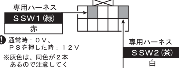
エンジンスイッチの裏側 10P白色カプラ
