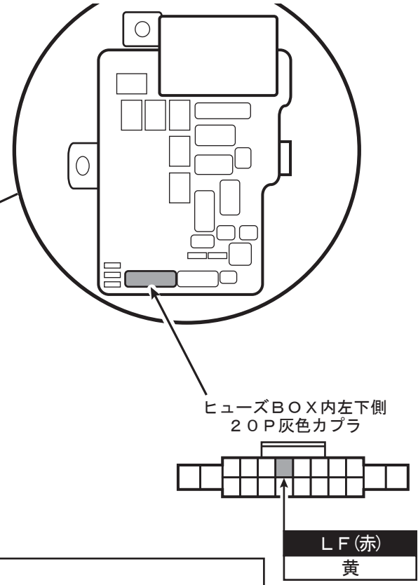
ヒューズBOX拡大図(表側)
