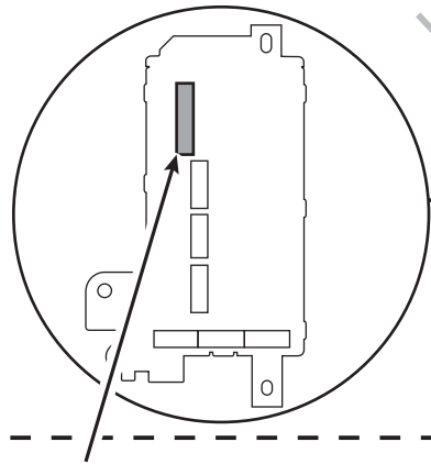
ヒューズブロック裏側の 右上側 40P白色カプラ
