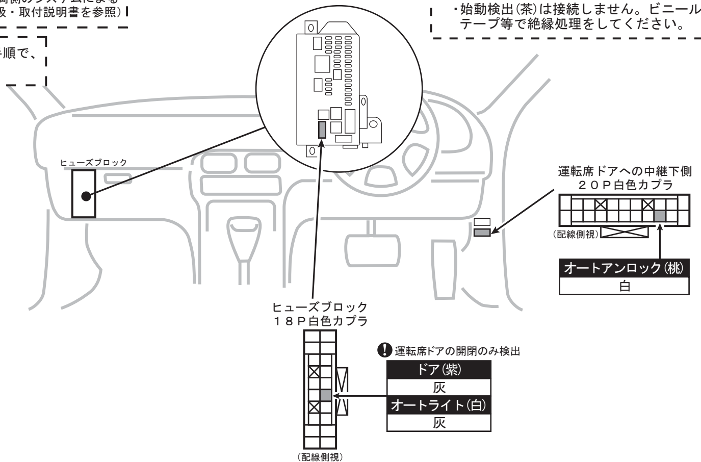
ヒューズブロック拡大図
