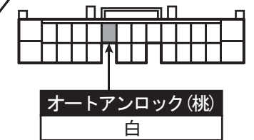
運転席ドアへの中継下側 26P白色カプラ
