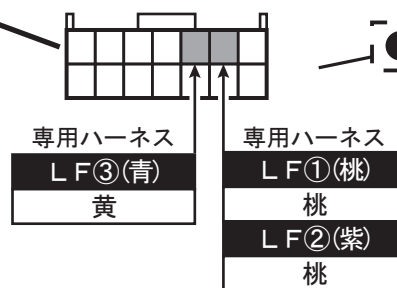
サイドカバー内 下側中継 14P白色カプラ
