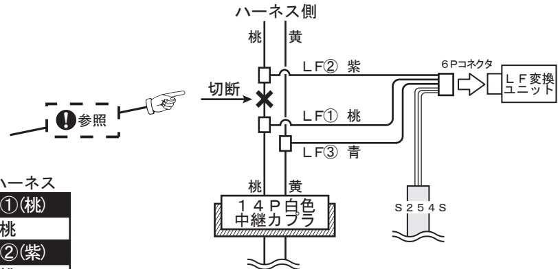
サイドカバー内 下側中継 14P白色カプラ
