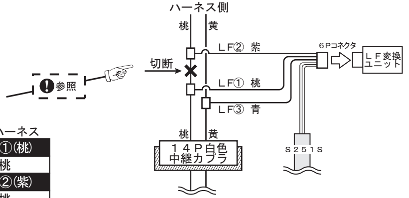
サイドカバー内 下側中継 14P白色コプラ
