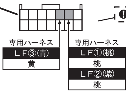
サイドカバー内 下側中継 14P白色コプラ
