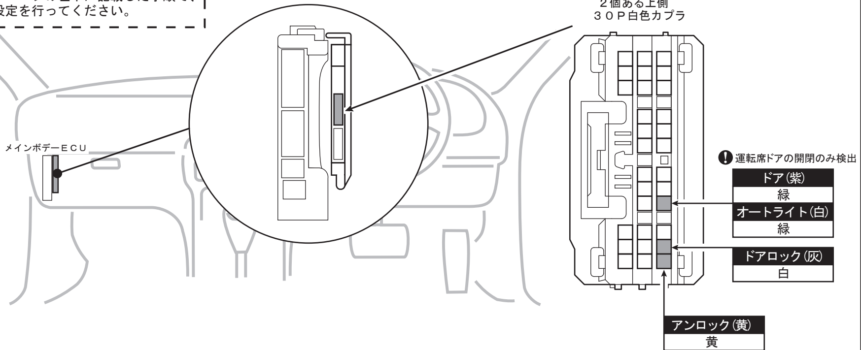
メインボデーECU拡大図
