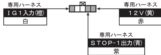
フットブレーキの奥側 5P白色カプラ
