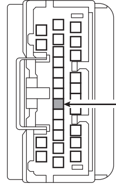
スマートキーコンピュータASSY 上から2番目 27P白色カプラ
