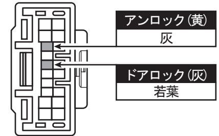
サイドカバー内左上側 18P白色コネクタ
